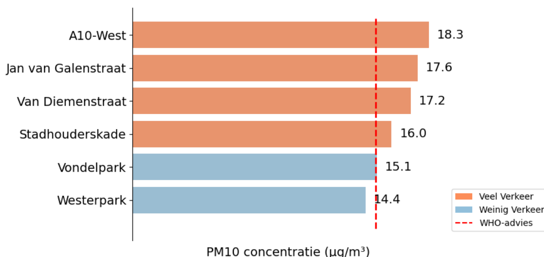
Figuur 4 Jaargemiddelde PM 10 concentratie
