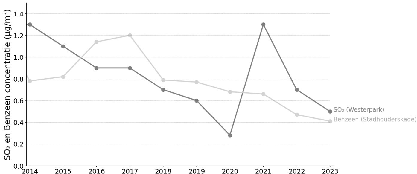
Figuur 18 Trend jaargemiddelde benzeen en SO 2 concentratie in de afgelopen 10 jaar
