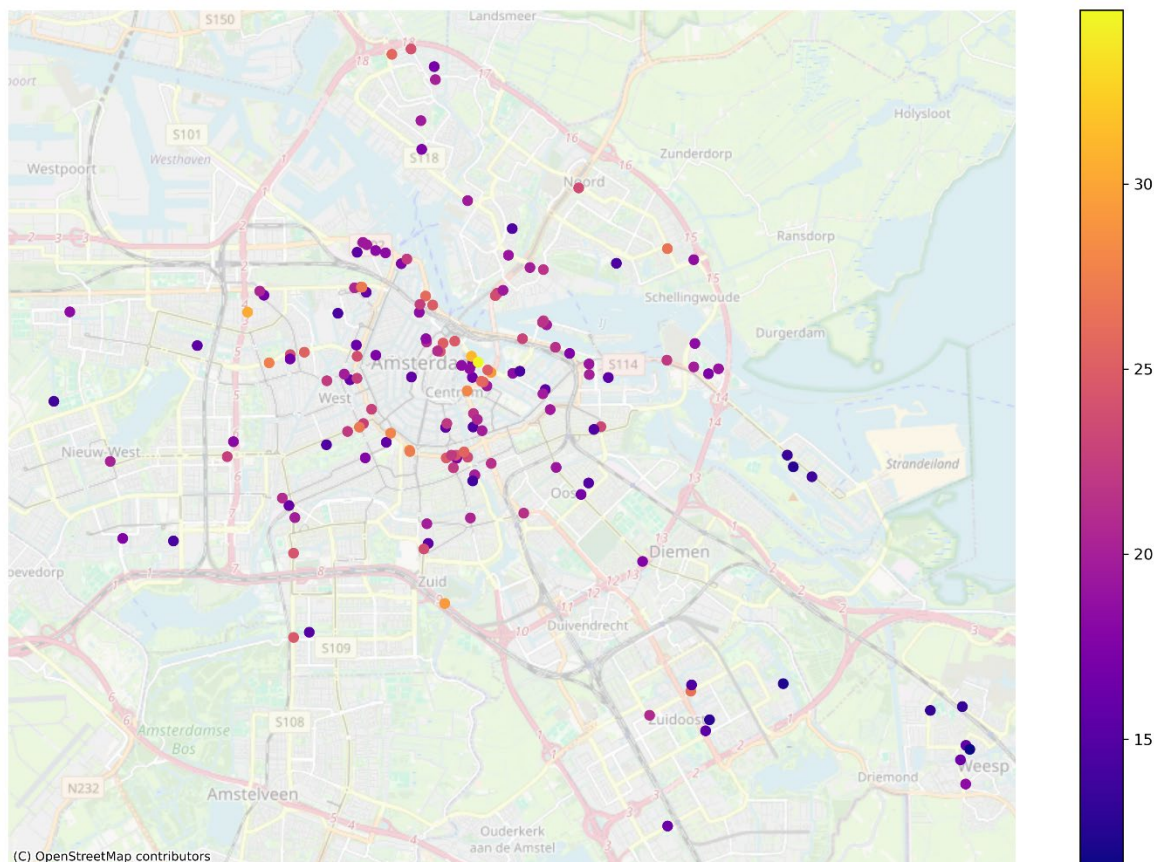
Figuur 3 Locaties en concentratie ( \mu\text{g}/\text{m}^3 ) NO 2 -Palmesbuisjes 2023
